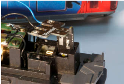
5. Neue LED-Leiterplatte leicht schräg einführen.
