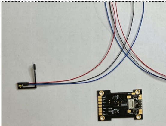
1 Stk. Multifunktions-Platine (Lokdecoder) 1 Stk Innenbeleuchtungs-Platine 2 Stk. Frontlicht-Platinen
