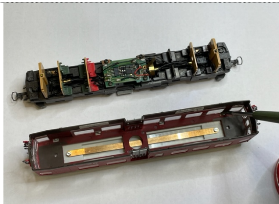
Dachteile vorsichtig mit Schraubenzieher (Keilklemme) aushebeln.
