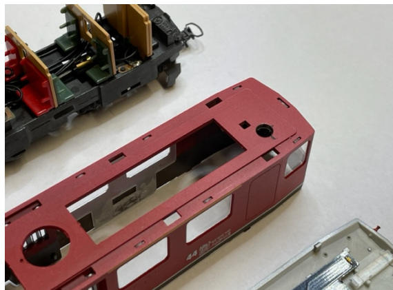
Abbildung der gebohrten Führerstandbeleuchtung.
